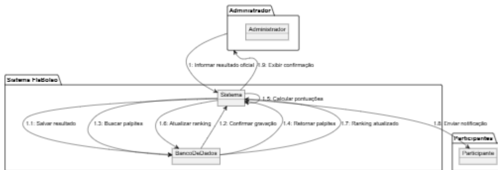
Diagrama de Comunicação - UC-11 Registrar Resultado da Partida
