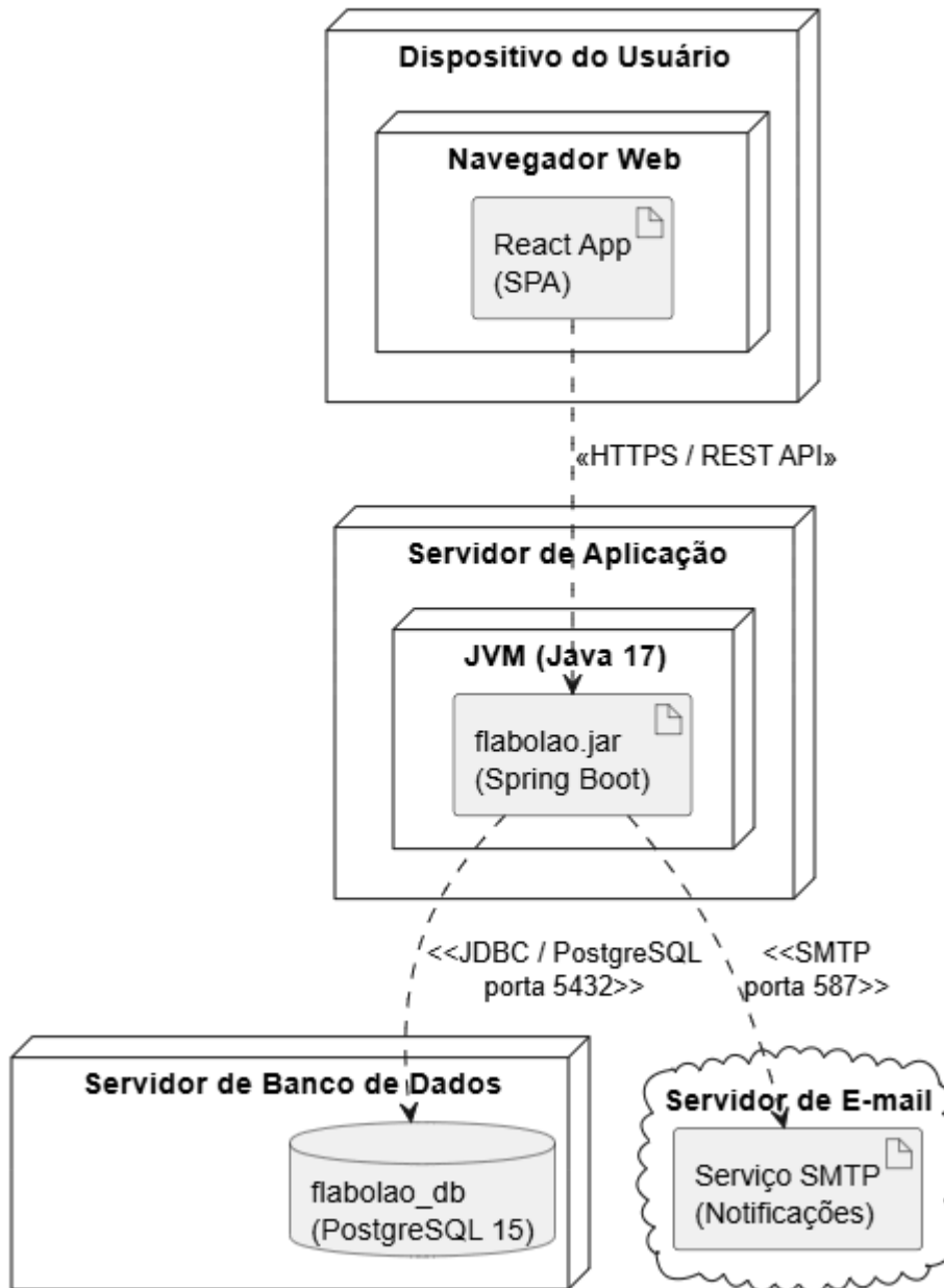
Diagrama de Implantação - Sistema FlaBolão
