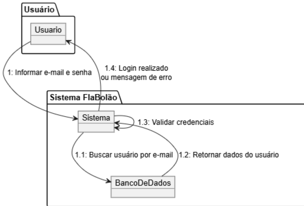
Diagrama de Comunicação - UC-02 Realizar Login
