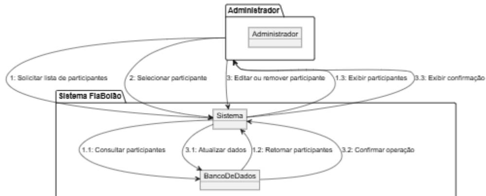
Diagrama de Comunicação - UC-03 Gerenciar Participantes
