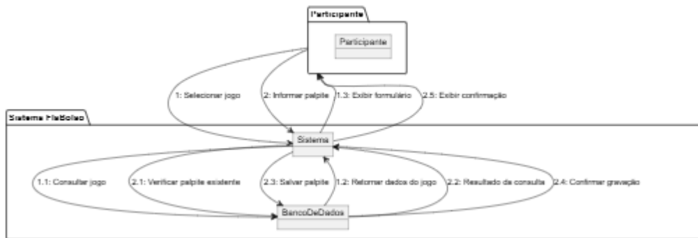
Diagrama de Comunicação - UC-08 Registrar Palpite
