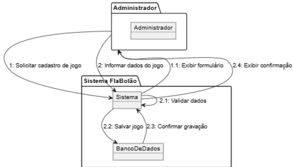
Diagrama de Comunicação - UC-04 Cadastrar Jogo
